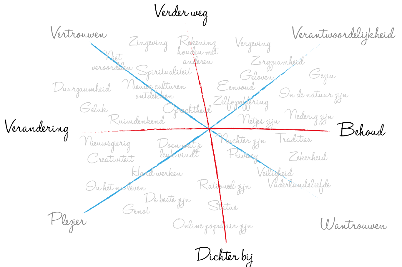
Waarden op de twee assen van het waardenmodel
